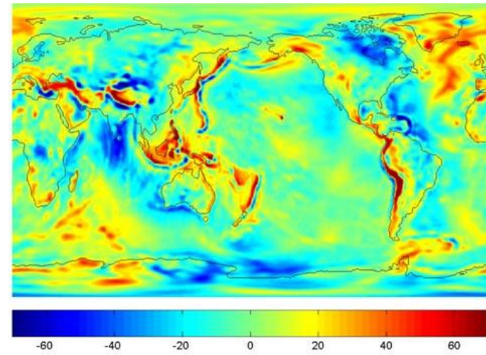
Модель глобального гравитационного поля GGMO2S, полученная за 1 год работы системы Grace
