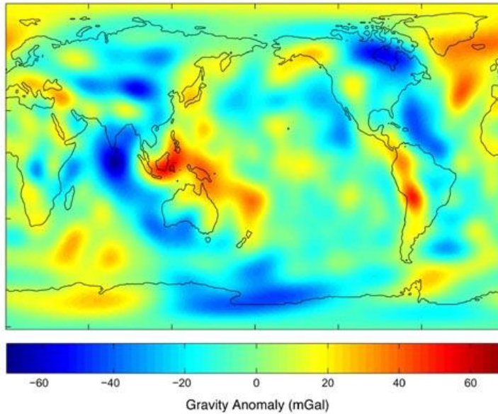
Глобальное гравитационное поле, полученное за 10 лет слежения за орбитами спутников.
